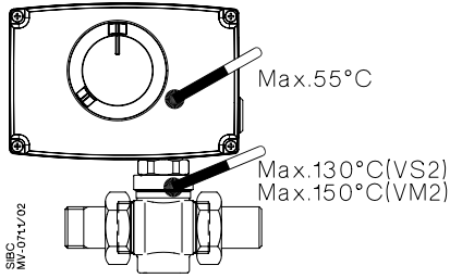
AMV 23, AMV 33 + VM2, VS2
