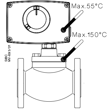
AMV 23, AMV 33 + VB2
